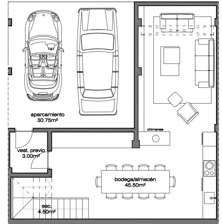
planta sótano
