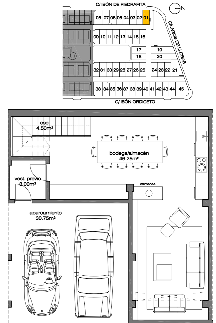
planta sótano
