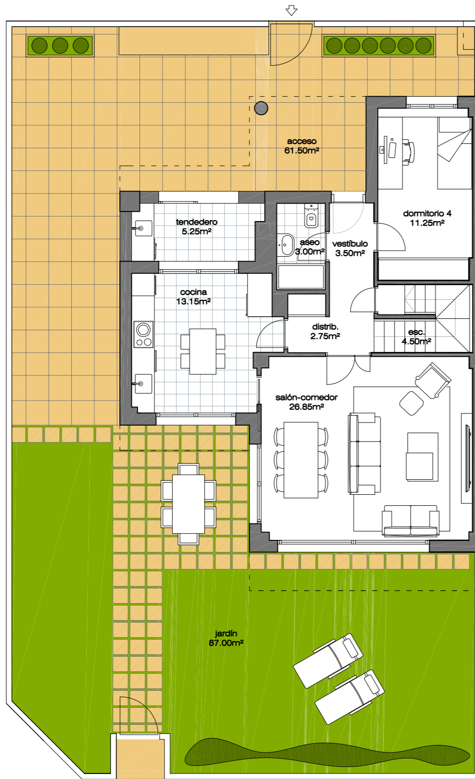
planta baja
