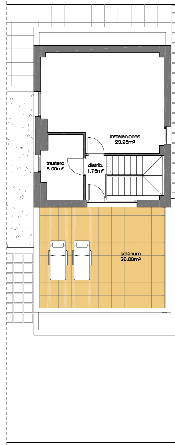
planta ático
