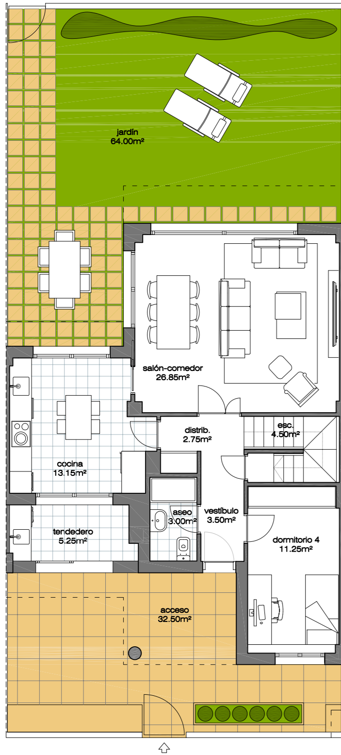
planta baja
