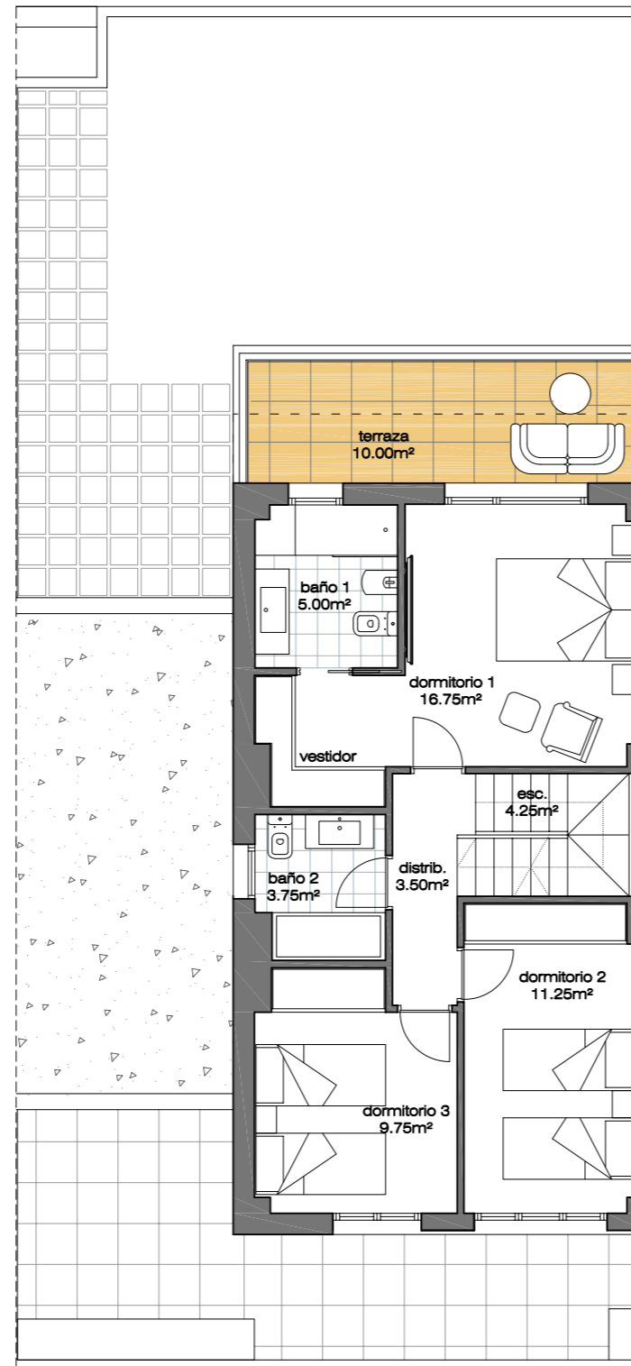
planta primera
