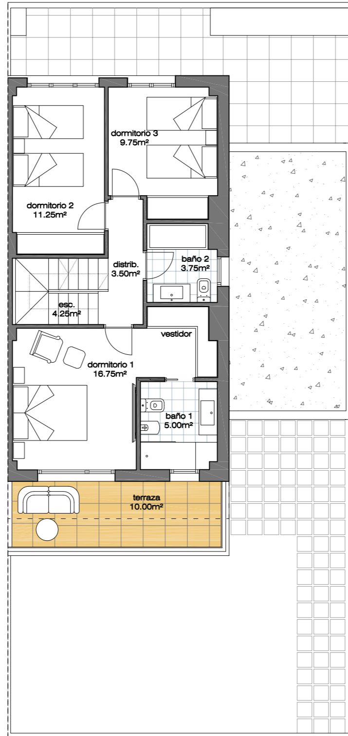
planta primera
