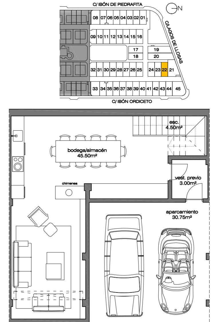
planta sótano
