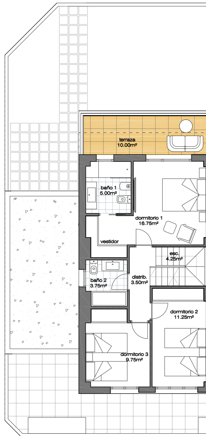
planta primera
