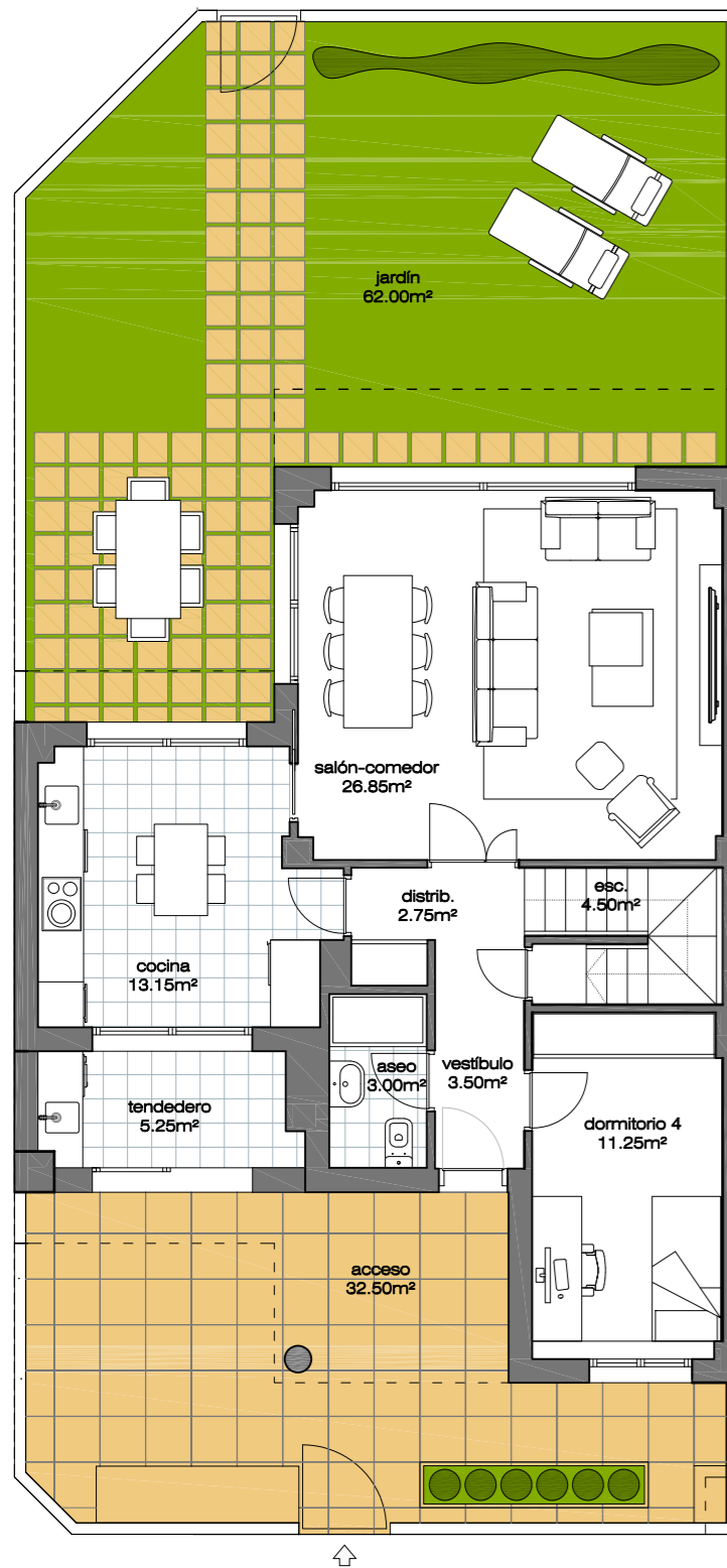
planta baja
