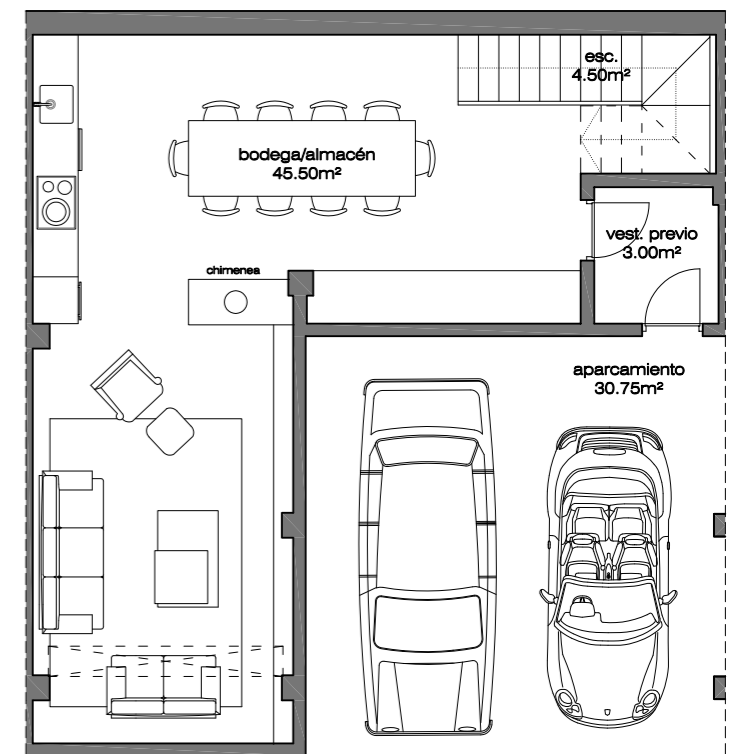
planta sótano
