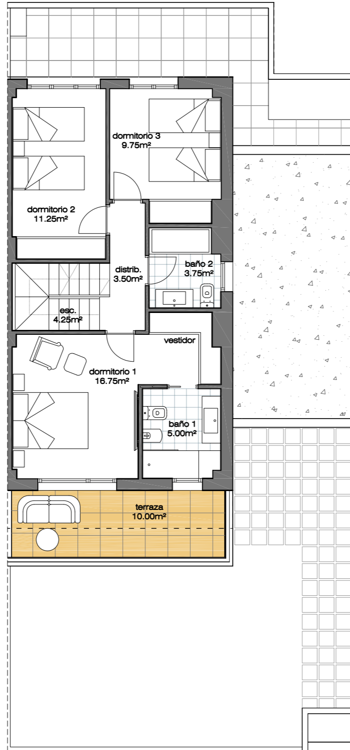
planta primera
