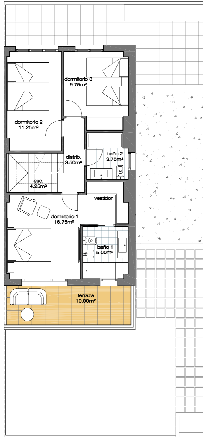
planta primera
