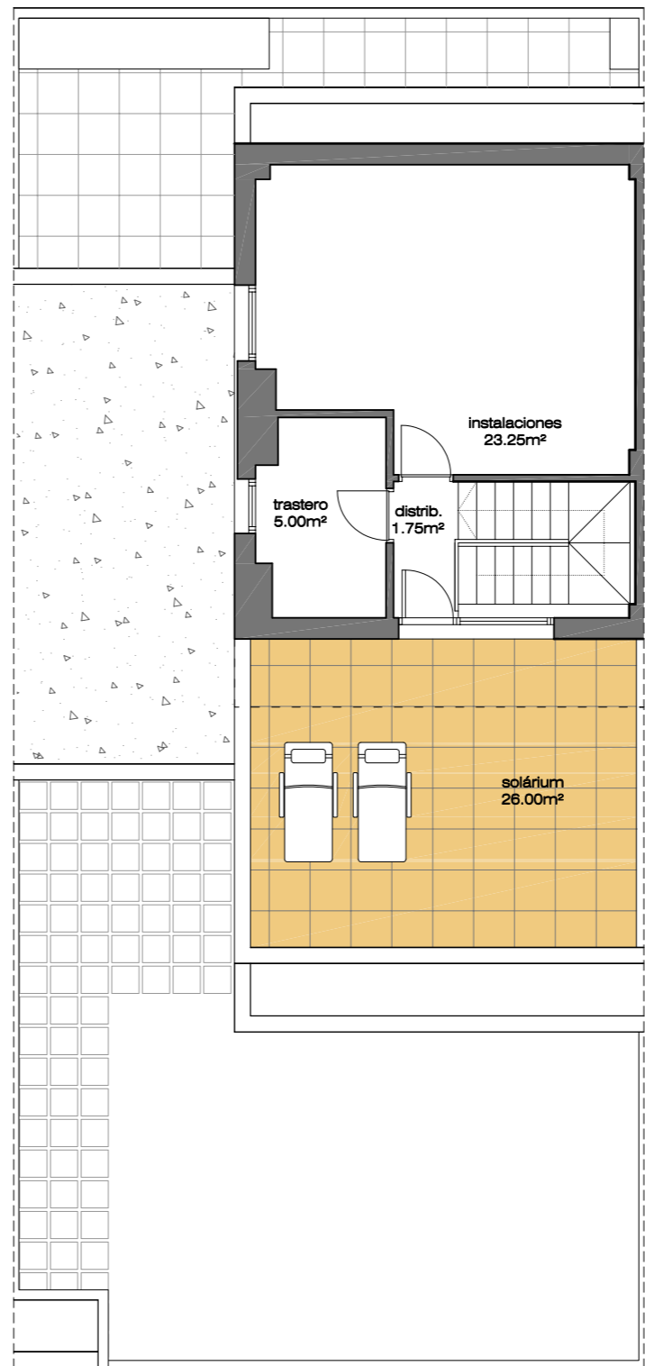
planta ático
