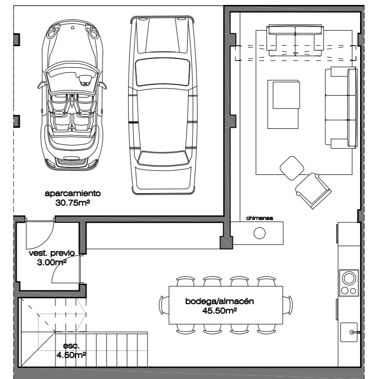
planta sótano
