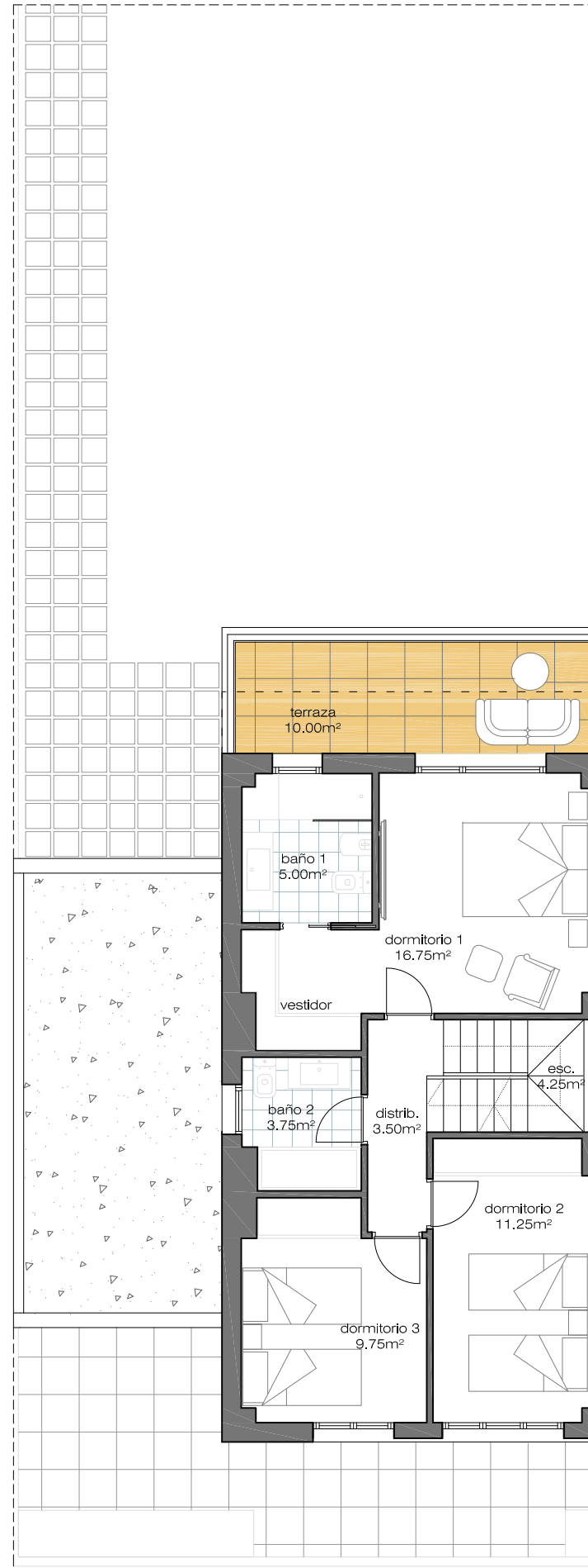
planta primera
