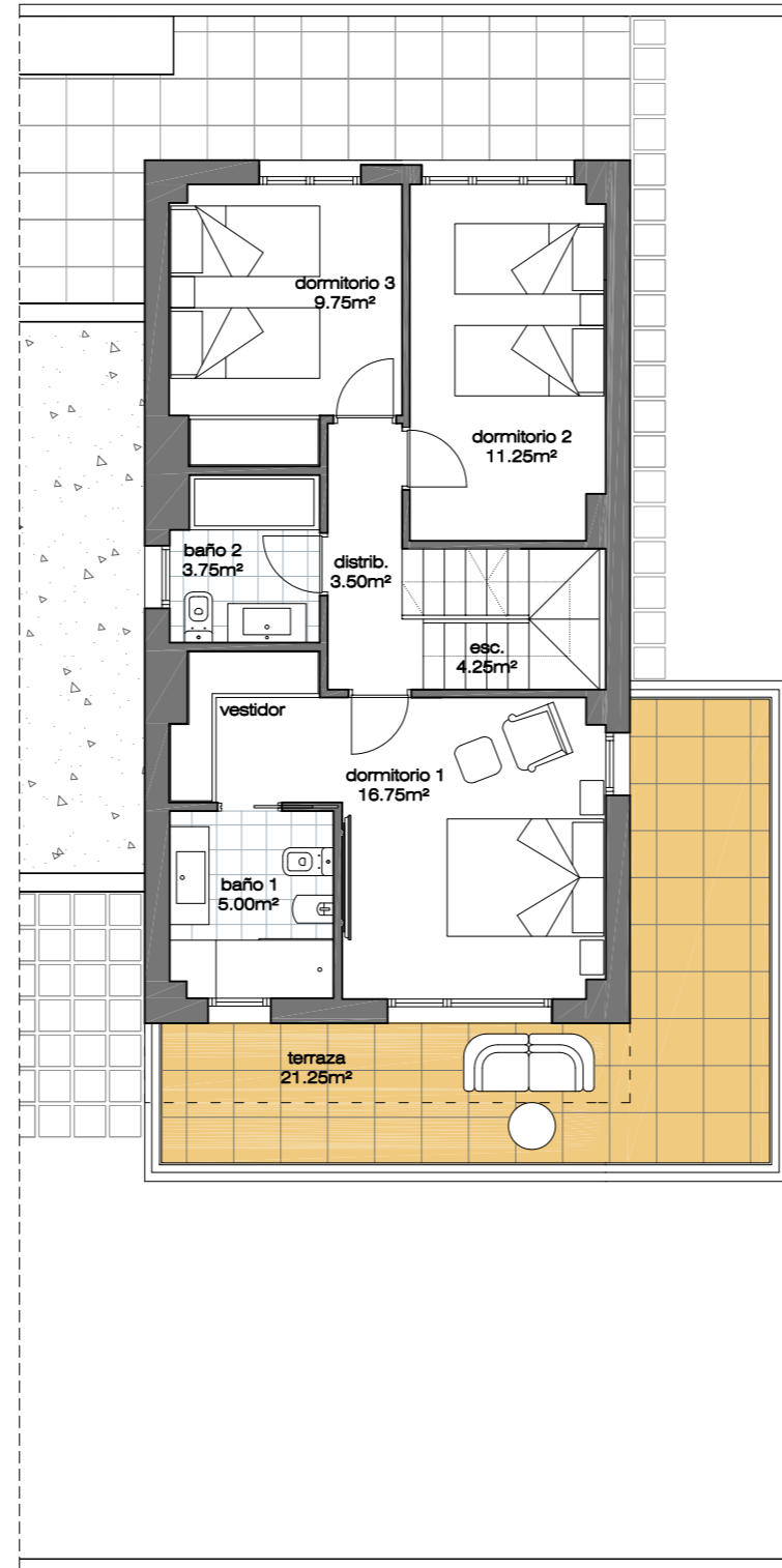
planta primera
