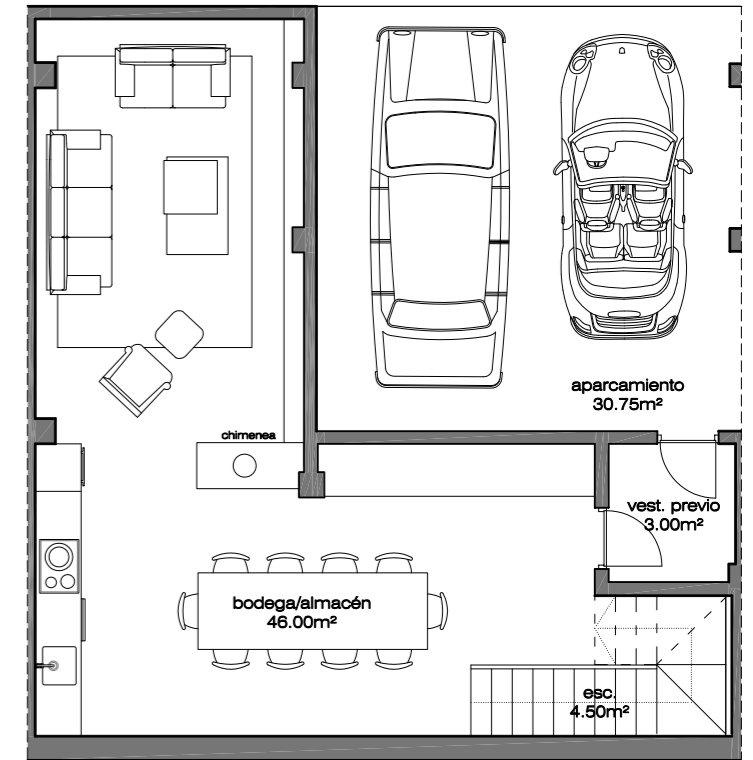
planta sótano
