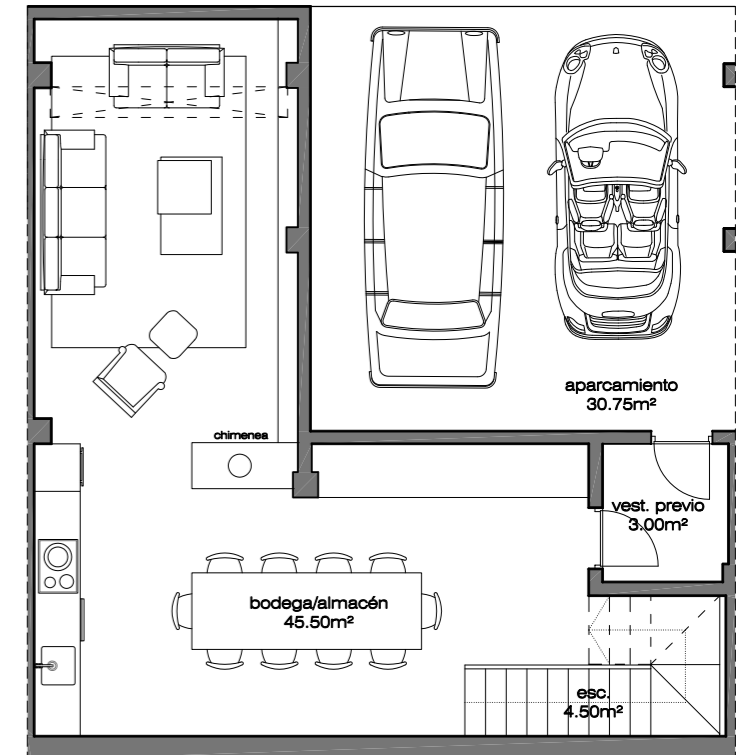
planta sótano
