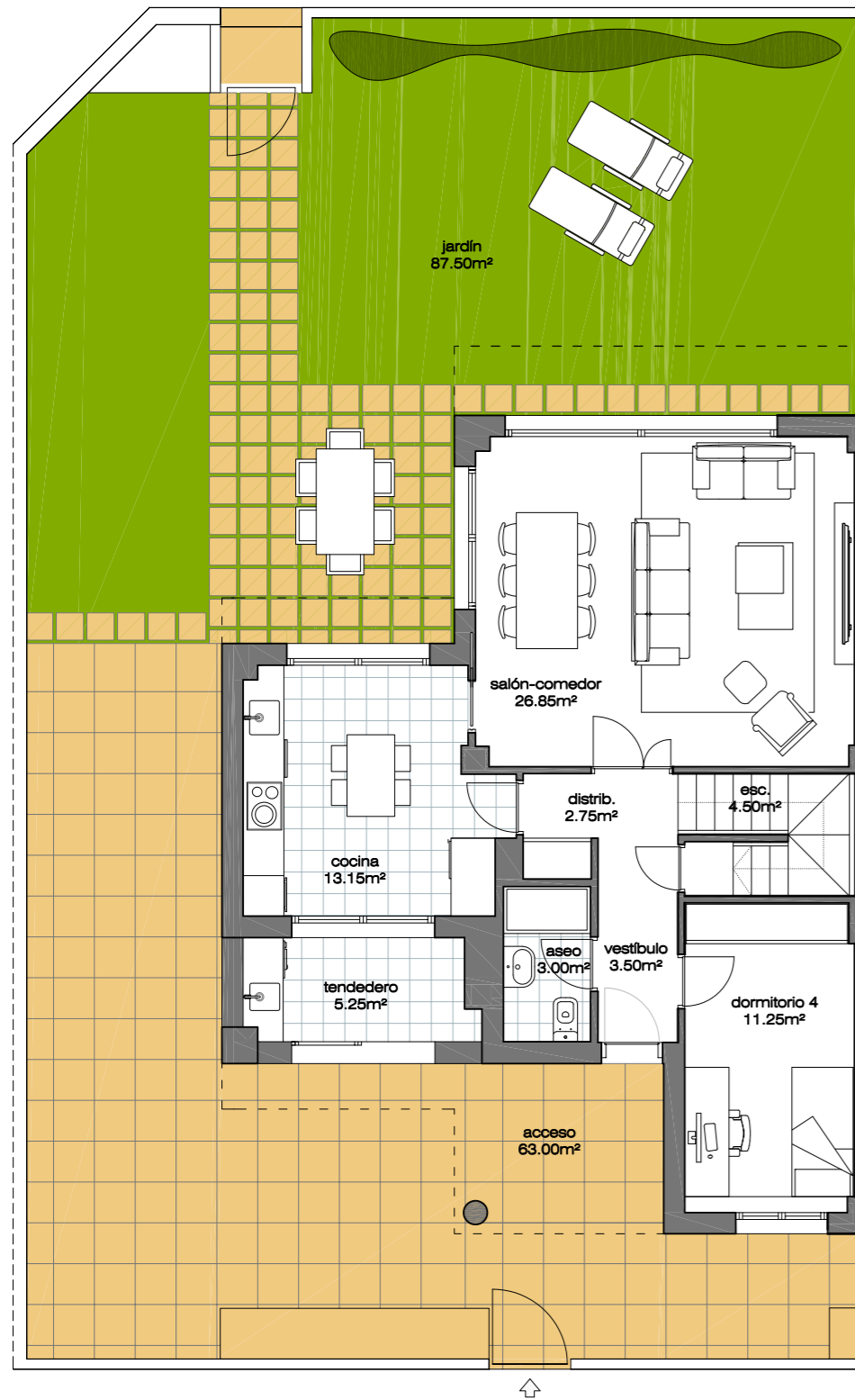
planta baja
