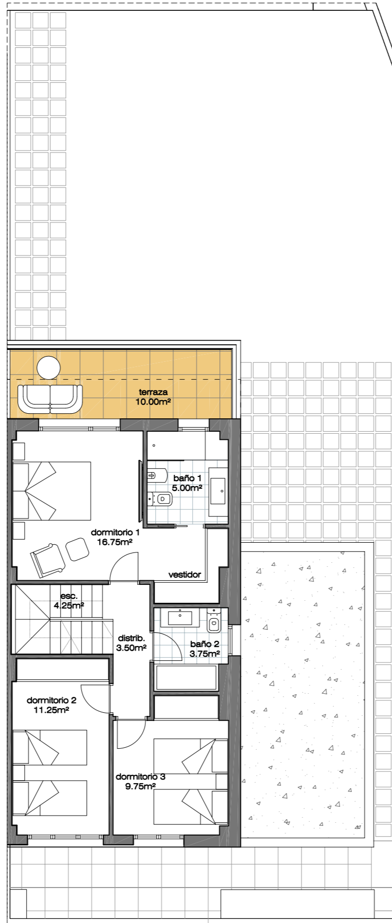
planta primera
