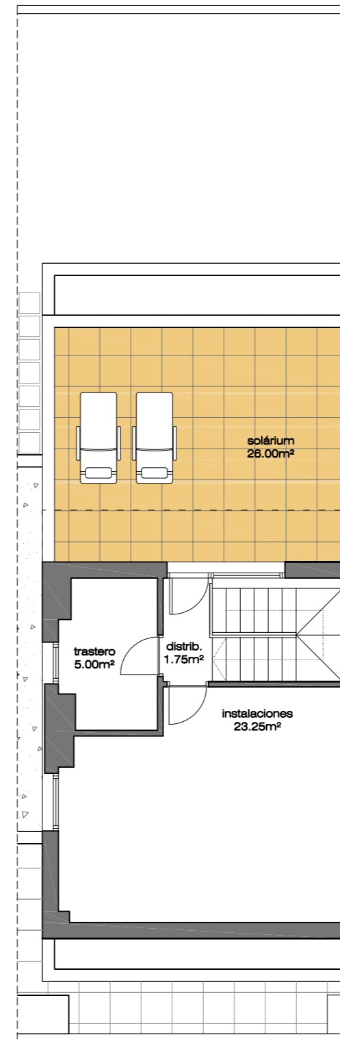
planta ático
