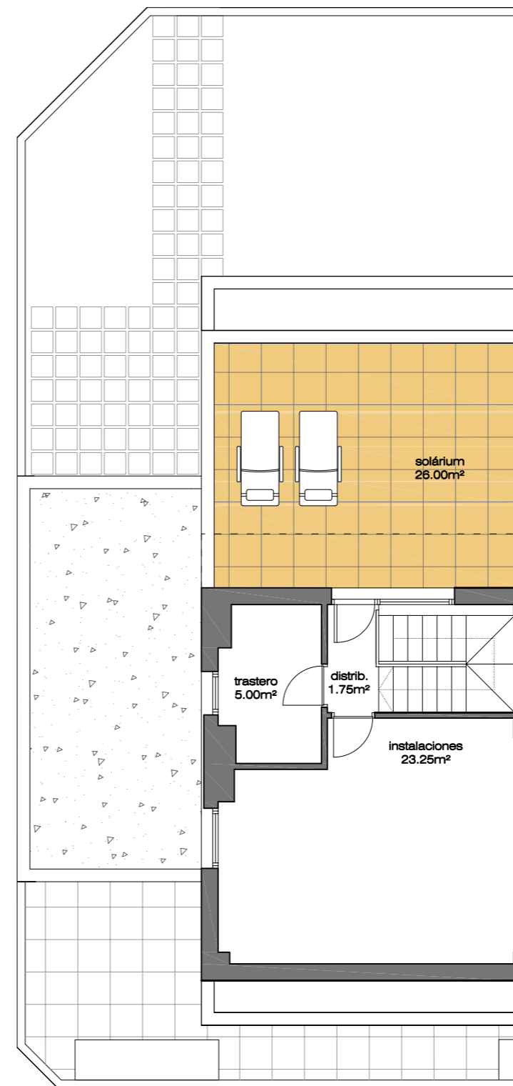
planta ático
