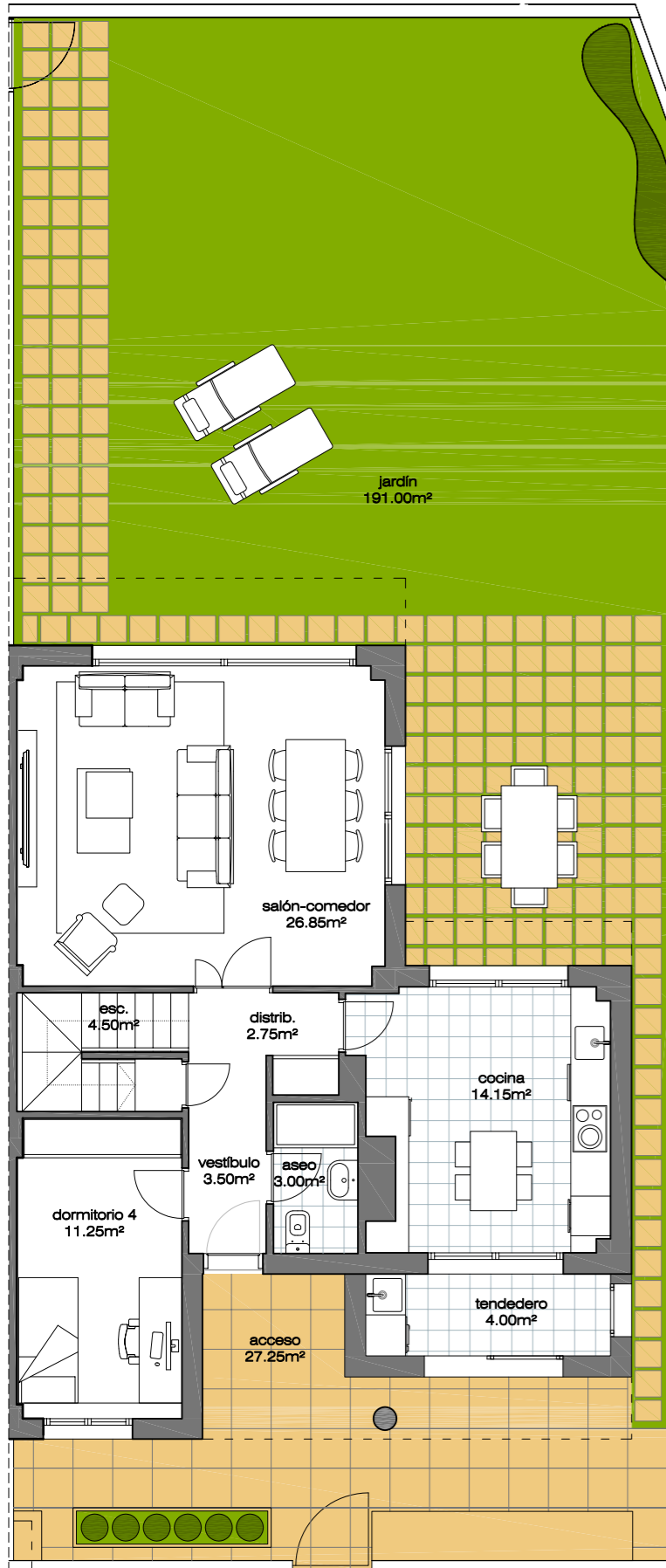
planta baja
