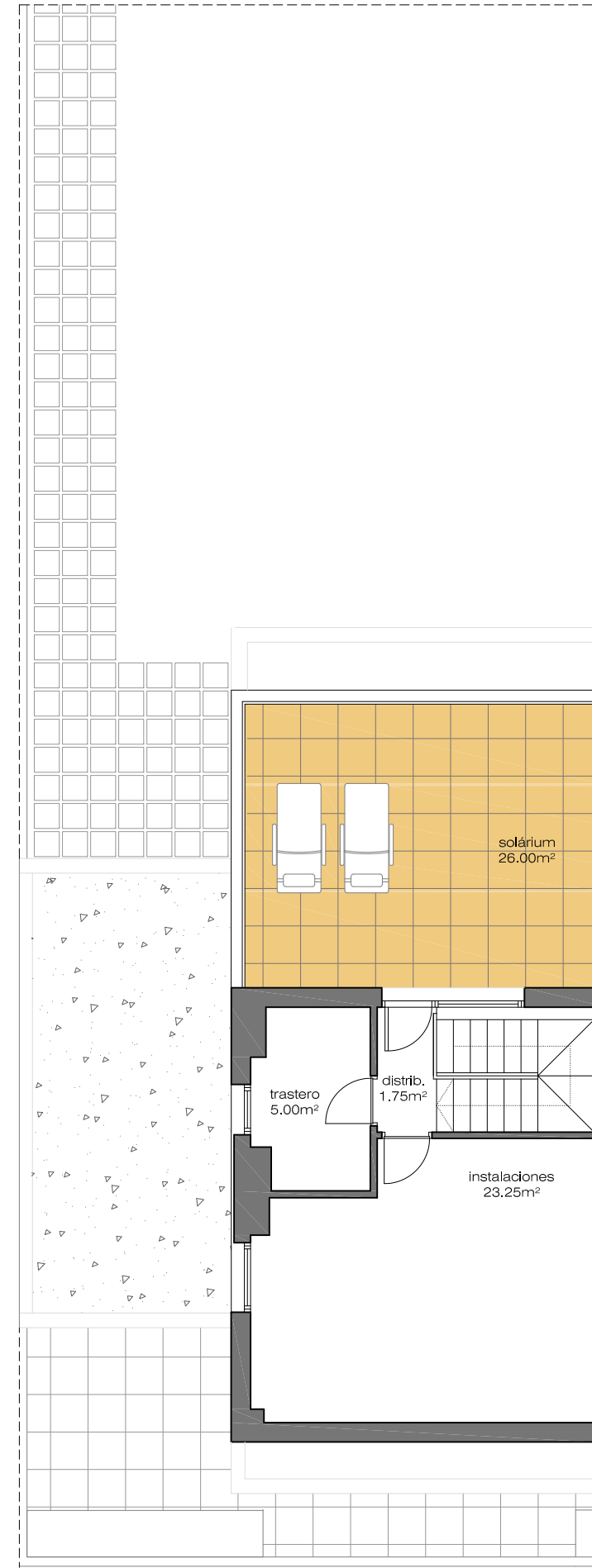
planta ático
