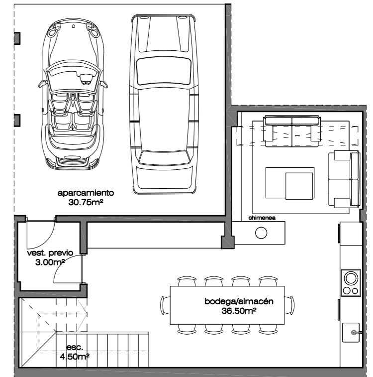
planta sótano
