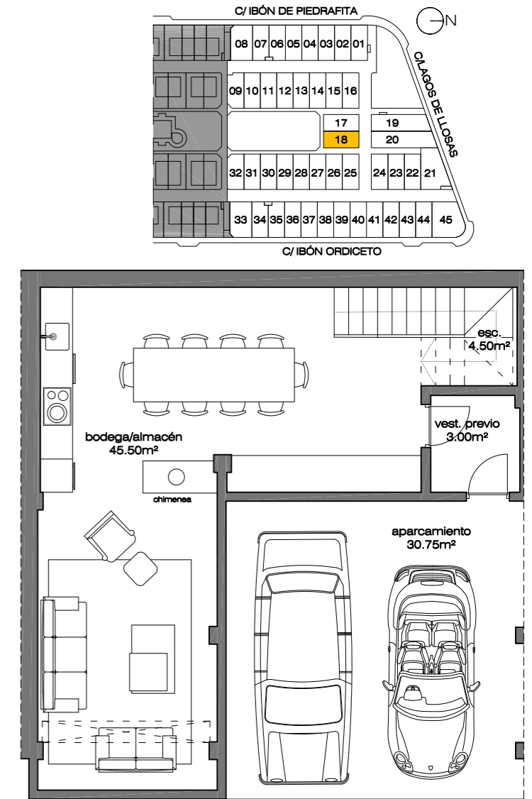
planta sótano
