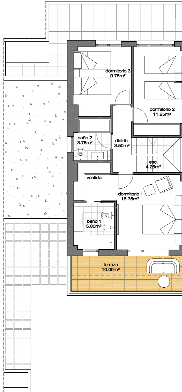
planta primera
