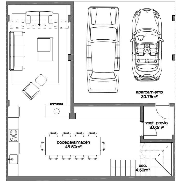
planta sótano
