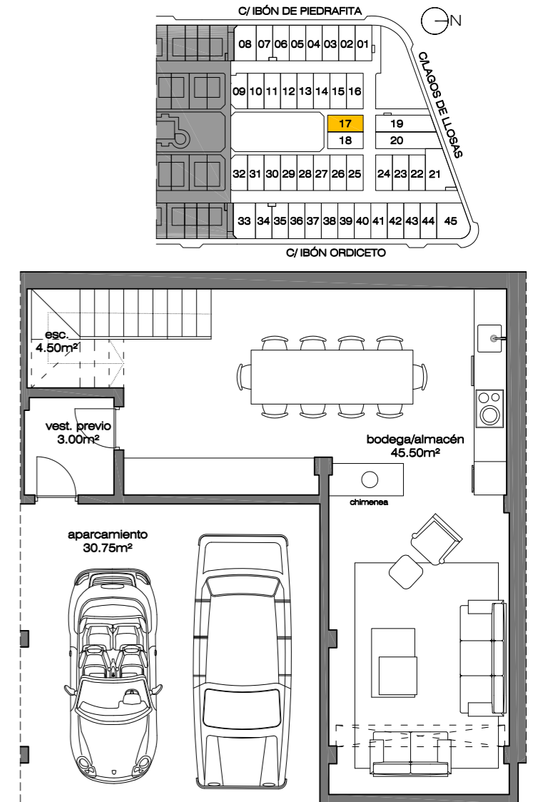
planta sótano
