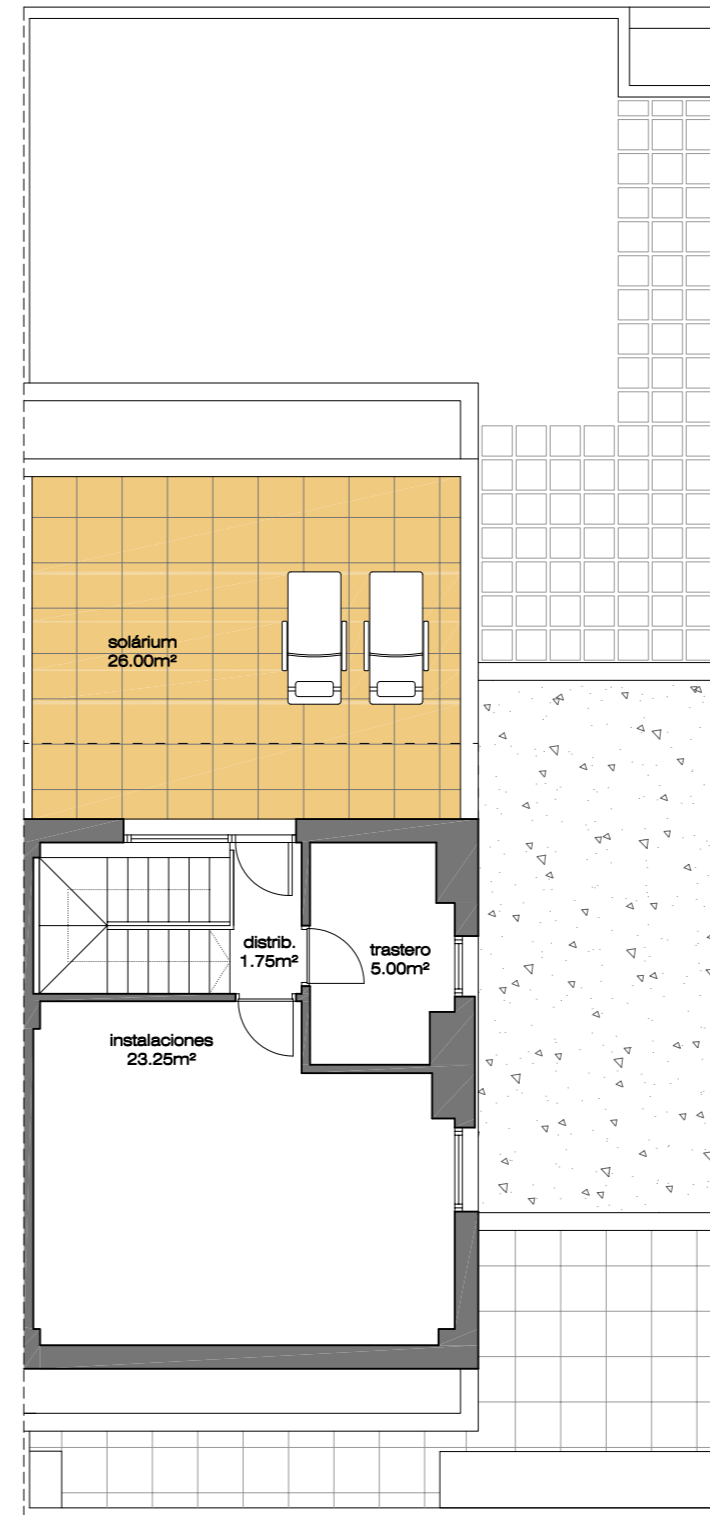
planta ático
